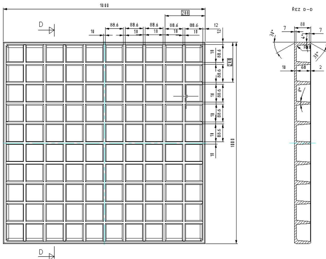
Obrázek 5: Sťěnový prvek MODUL 20 (forma Haselbeck)
